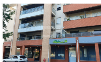
APARTAMENTO T3 Calendário, Famalicão
