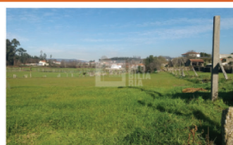
TERRENO URBANO Lemelhe, Famalicão
