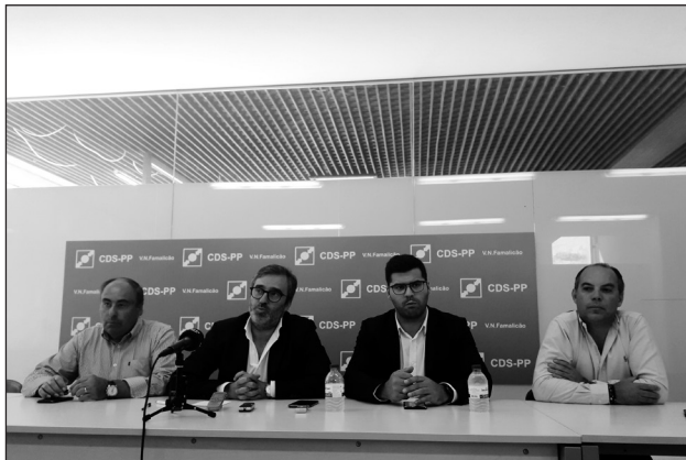
Centristas analisam resultados e projectam o futuro
